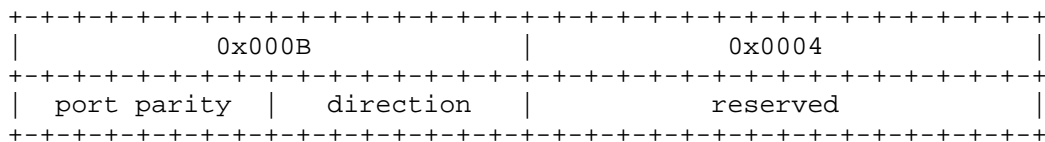
Figure 14: PER parameter set attribute
